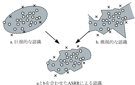
図 4: ASRR による認識 (○ は正事例、× は負事例)
