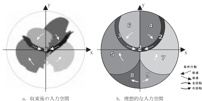
図 8: 左車輪の回転速度が 15\% 低下した場合
