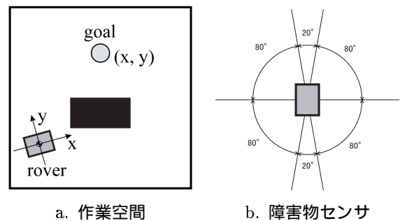
図 9: 問題設定
